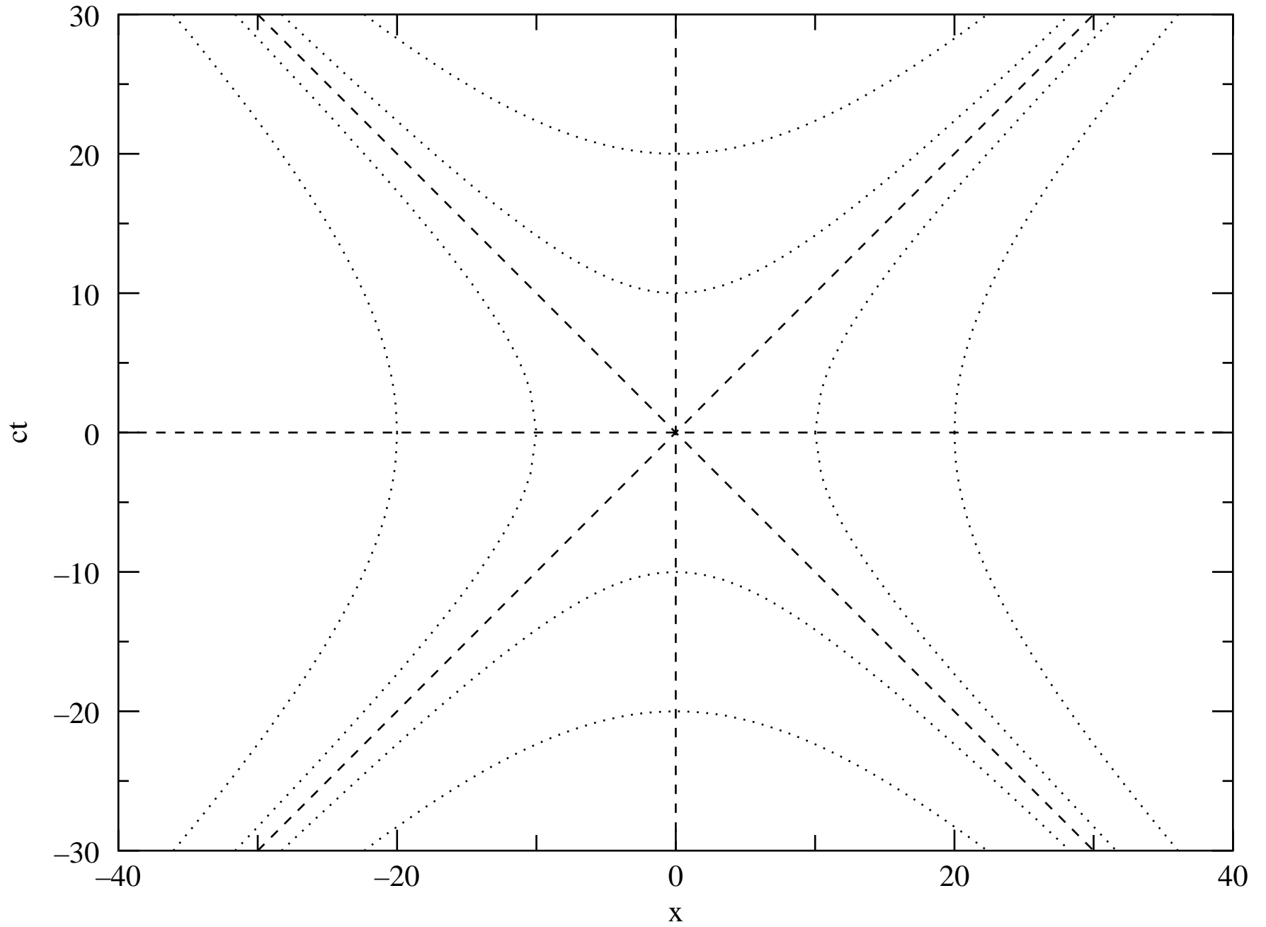
Minkowski Diagram
